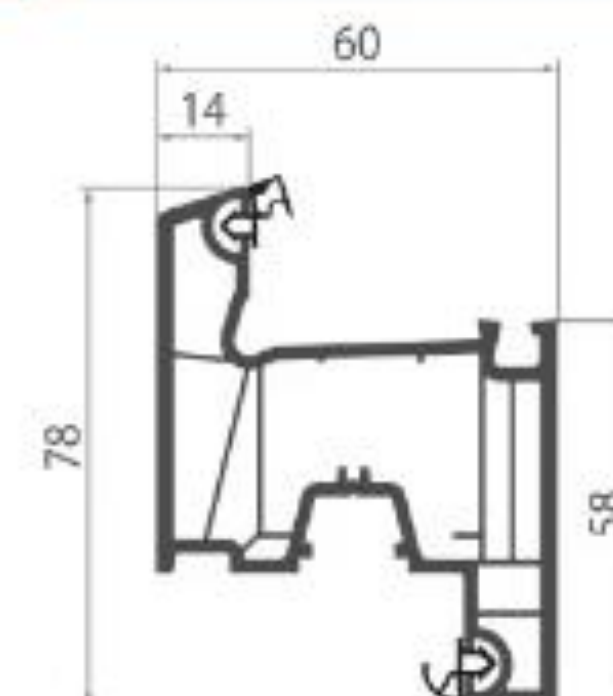
012 Stulp
