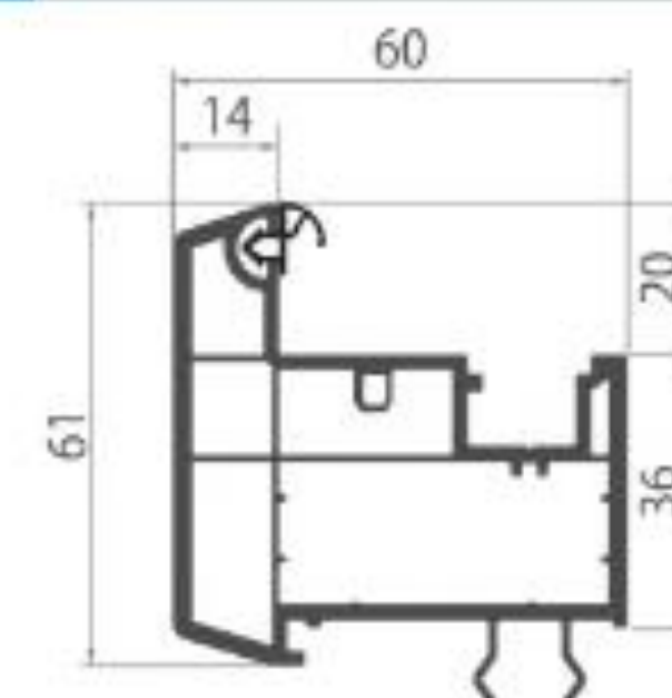
012 Stulp
