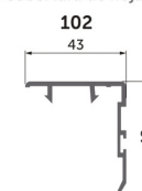
Cover profile for sash SL 39/90 Perfil de cobertura de hoja SL 39/90
