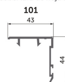
Cover profile for sash SL 39/82 Perfil de cobertura de hoja SL 39/82
