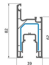
Sash SL 39/82 Hoja SL 39/82 098
