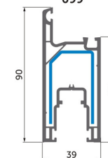
Sash SL 39/90 Hoja SL 39/90 099
